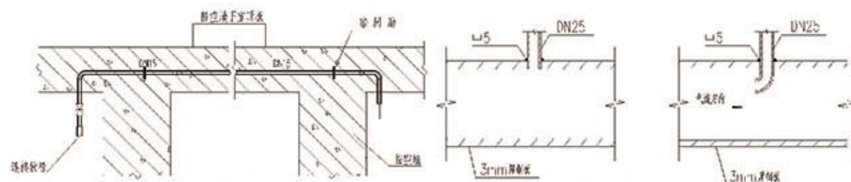
测压管安装示意图
