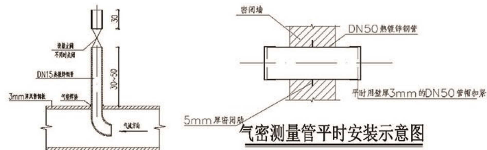
尾气监测取样管与风管连接示意图
