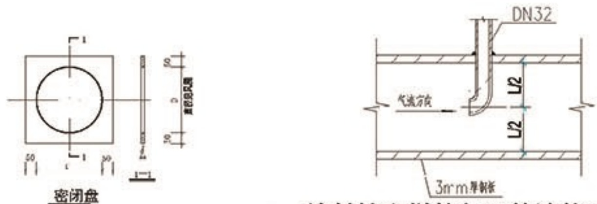
穿密闭墙短管及手动密闭阀连接法兰制安大样
