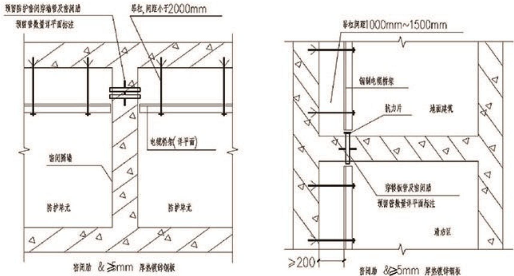
电缆桥架穿越密闭隔墙、楼板
