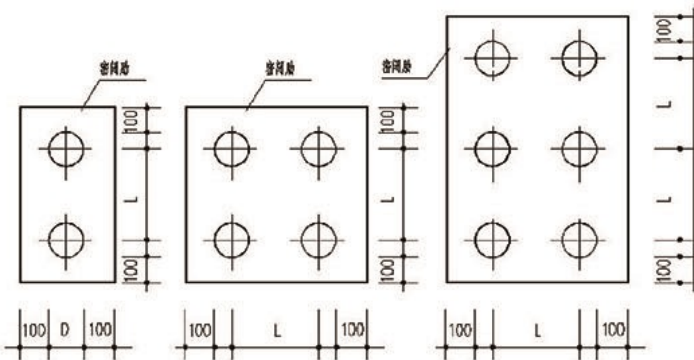
热镀锌钢管和密闭肋尺寸表
