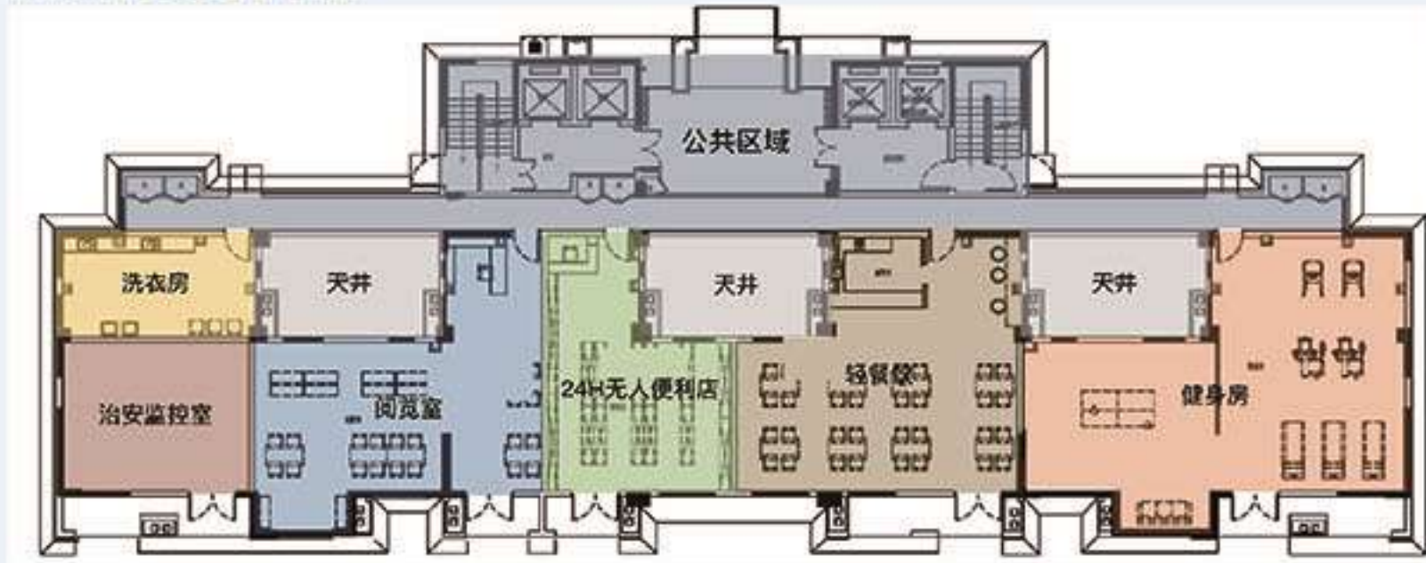
一层平面 FIRST FLOOR PLAN
